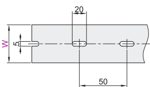
W < 80mm线槽底部孔尺寸
