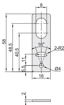
直角安装 ZLP12
