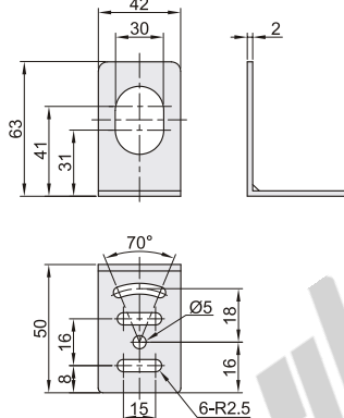
规格: M30
