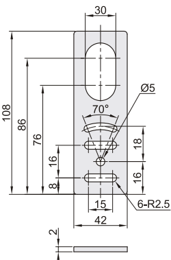
规格: M30
