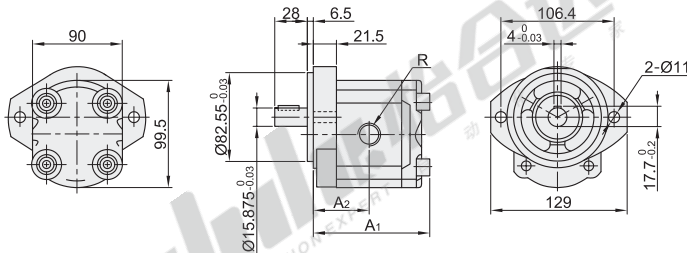
标准齿轮泵 WSN32 规格: 3A
