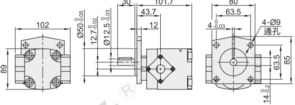
标准齿轮泵 WSN32 规格: 2A
