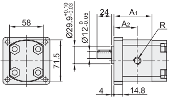
标准齿轮泵 WSN32 规格: 1A
