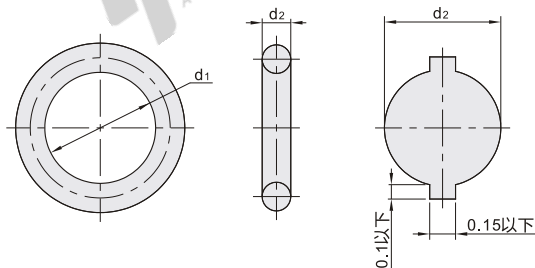
① 截面放大图
