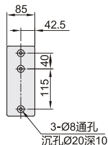
■ 安装板尺寸
