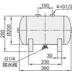
底架安装孔尺寸
