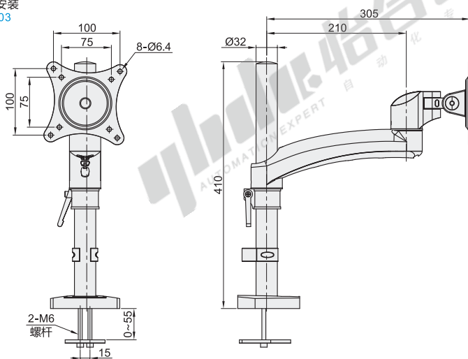
穿孔安装 NHD03
