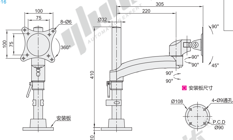
锁孔安装 NHD16
