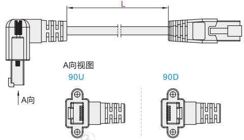
直角型 NHN53/54
