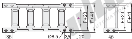
桥式 VEY71
