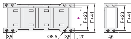
封闭式 VEY73
