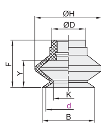
盘径Ø10~50
