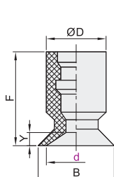
平形 盘径Ø2~8
