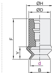
风琴形 盘径Ø6~8
