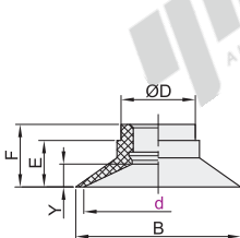
平形 盘径Ø10~50
