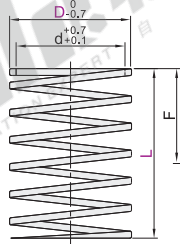
最大压缩量50%(深紫色)
