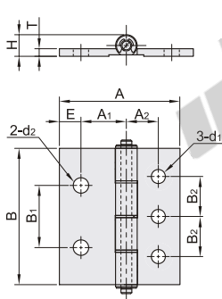
圆孔型 HFC96
