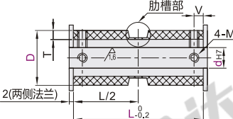
带法兰型 ENK23/24
