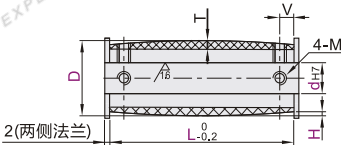
带法兰型 ENK13/14
