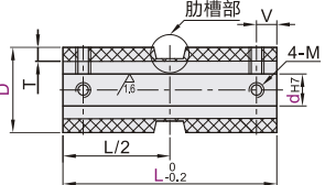
无法兰型 ENK21/22
