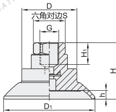
内接螺纹 外形B
