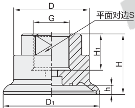
内接螺纹 外形A
