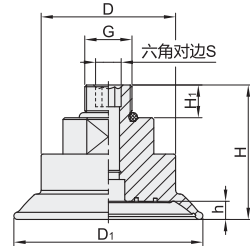
外接螺纹
