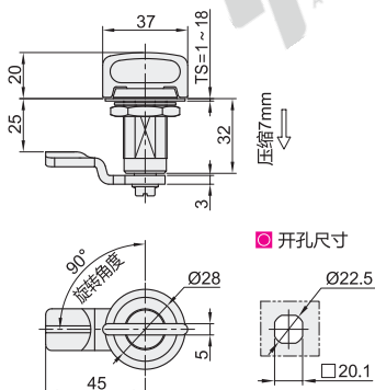
30系列·止口高度25 XAS52
