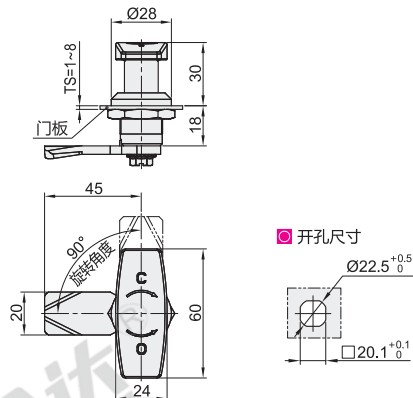
60系列·止口高度18 XAS51
