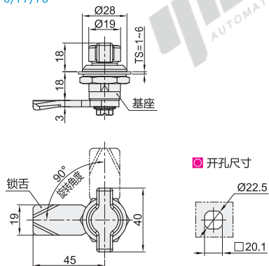
40系列·止口高度18 XAS75/76/77/78
