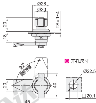
40系列·止口高度18 XAS53
