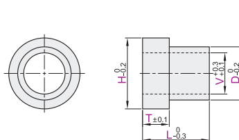
肩型 UCM51/52/56/57/66
