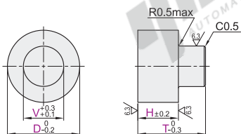
台阶型 UCM01/02/06/07/16
