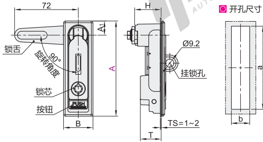
带锁芯带挂锁型 XAT18
