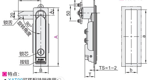
带锁芯带挂锁型 XAT09 带锁芯 XAT10
