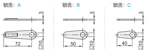
锁舌形状
