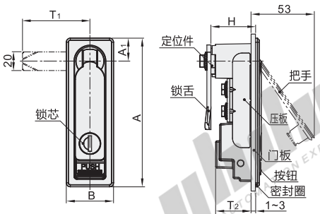
带锁芯 XAT11 XBT08 XBT09 XBT10
