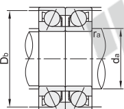
安装图
