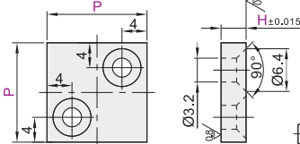
双孔方形 PHR11/12
