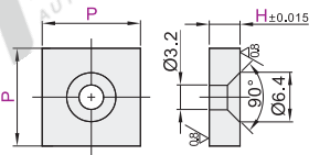
单孔方形 PHR06
