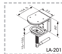
LA-528-1 Grommet Type
