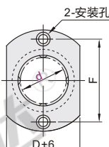
对边法兰型 E-LMF21/22
