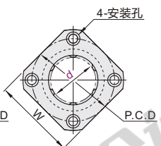
方法兰型 E-LMF11/12
