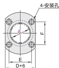
对边法兰型 E-LMF21/22
