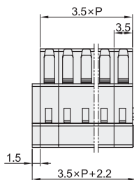
插座 ZKY10
