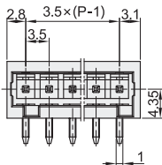
插头 ZKY09
