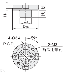
圆锥凸轮套 HCD13
