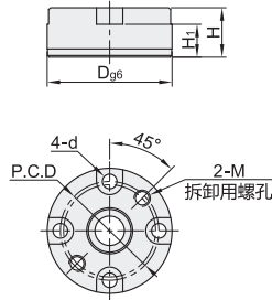
圆柱套 HCD12
