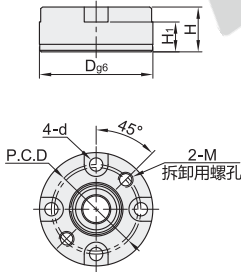
圆锥套 HCD11
