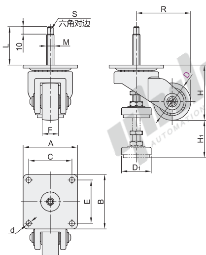
丝杆活动型(无刹)
