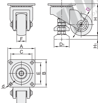
丝杆活动型(无刹)
