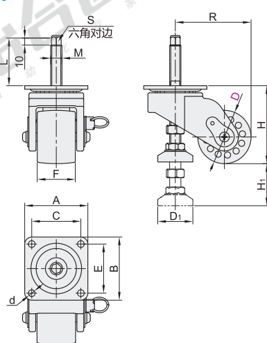
丝杆活动型(五金边刹)
