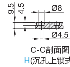
C-C剖面图 H(沉孔上锁式)
