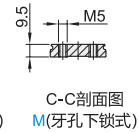
C-C剖面图 M(牙孔下锁式)
