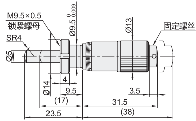
带锁紧螺母·球面测量面(SR4) EPF09-148-143
