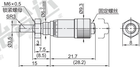
带锁紧螺母·球面测量面(SR3) EPF09-148-243
