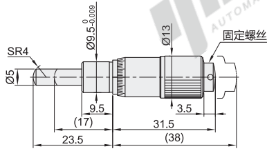
直柄型·球面测量面(SR4) EPF09-148-142
