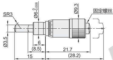
直柄型·球面测量面(SR3) EPF09-148-242
