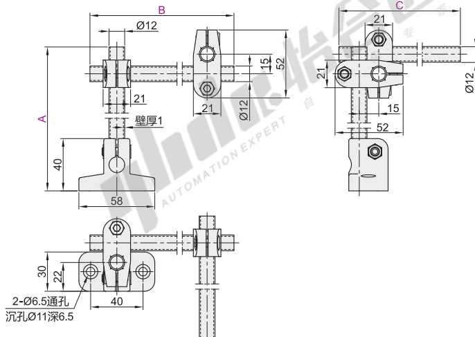
传感器安装块(标配件)
