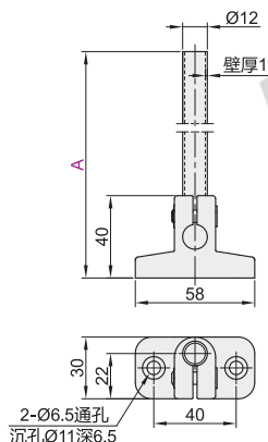
单管可调 ZLP34
