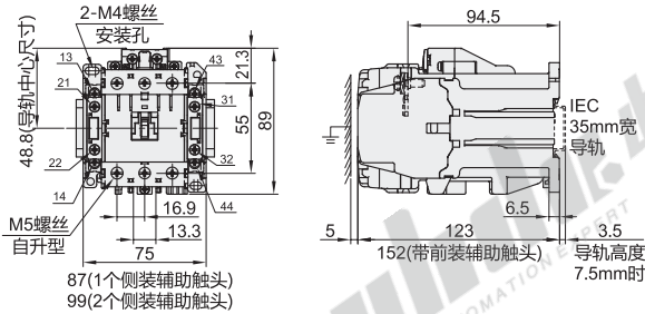
MS-T系列辅助触头
