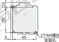
安装尺寸图
