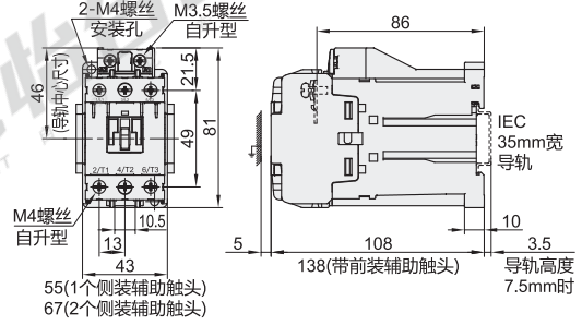
安装尺寸图
