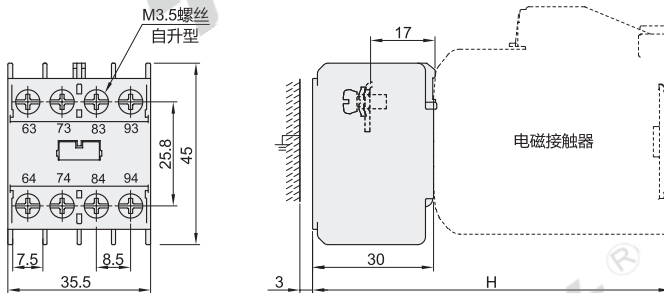
MS-T系列辅助触头
