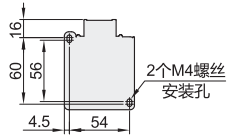
安装尺寸图
