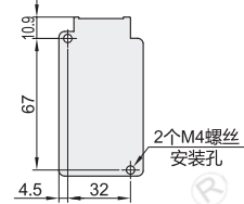
安装尺寸图
