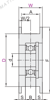
带法兰型 单轴承型 Y-EAF21
