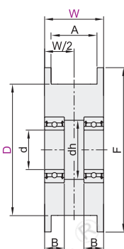
双轴承型 Y-EAF31
