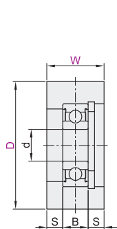
无法兰型 单轴承型 Y-EAF01
