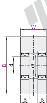
双轴承型 Y-EAF11
