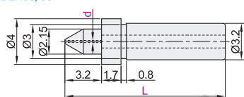
台阶型 BLN08/09
