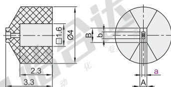
方孔形 BLN07
