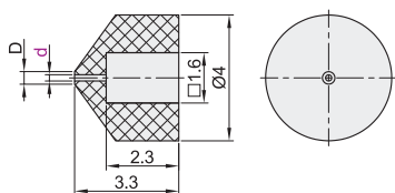
圆孔形 BLN06
