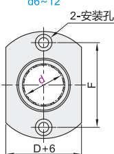
对边法兰型 Y-GVK41
