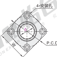
方法兰型 Y-GVK61
