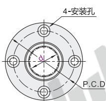
圆法兰型 Y-GVK51
