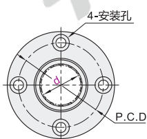
圆法兰型 Y-GVK21
