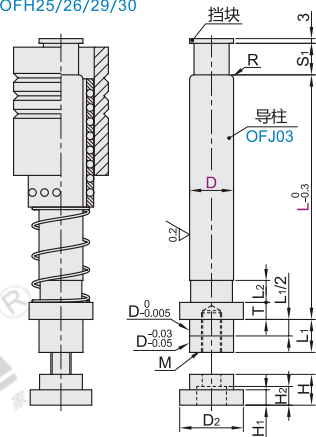
固定挡块 OFH25/26/29/30
