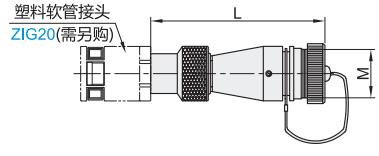
ZN(直式对接塑料软管插座)
