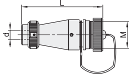
ZE(直式对接夹爪紧固插座)
