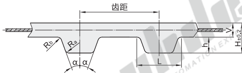
ECE22-MXL(齿距: 2.032)
