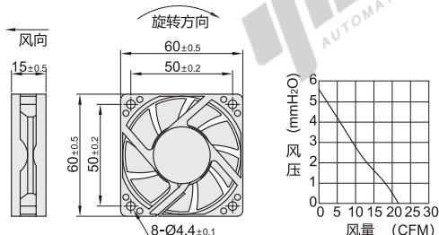
外形尺寸：6015M1
