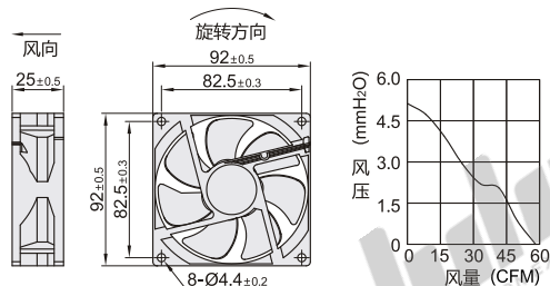
外形尺寸：9225M1
