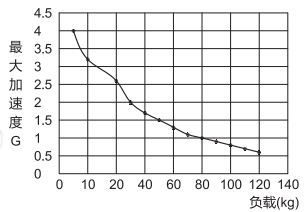
最大加速度VS负载
