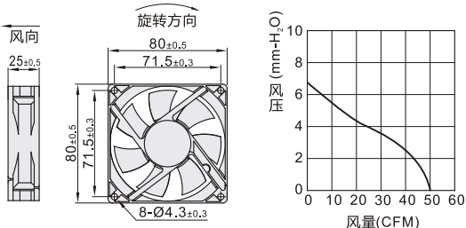
外形尺寸: 80
