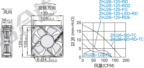
外形尺寸: 120
