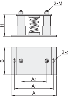
双弹簧型 NHF92
