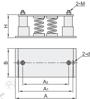
四弹簧型 NHF93
