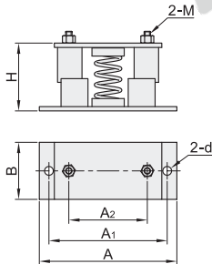
单弹簧型 NHF91
