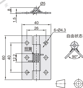
HFE66
