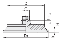
外接螺纹
