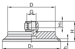
内接螺纹 外形B
