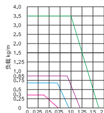
直线架空长度与负载关系图FLG 安全塌腰长度与负载关系图FLB
