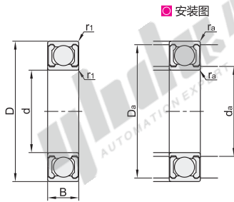
■ 安装图
