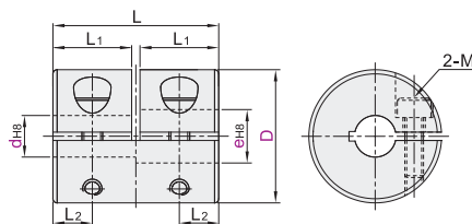
螺钉夹紧型 DEV12
