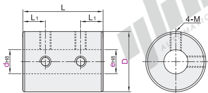
螺钉固定型 DEV02
