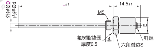
外螺纹短型·软管接头型 NHR37
