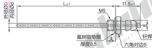
外螺纹短型·竹节接头型 NHR36
