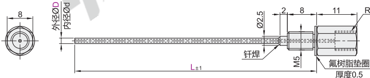
外螺纹长型·内螺纹 NHR24
