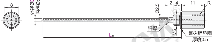
外螺纹短型·软管接头型 NHR37
