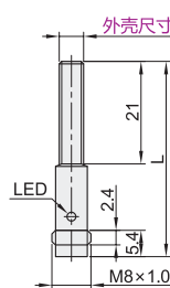
外壳尺寸：4/M5
