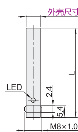
外壳尺寸：6.5
