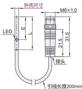
外壳尺寸：3
