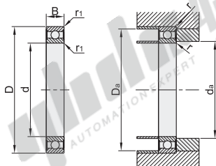
安装图
