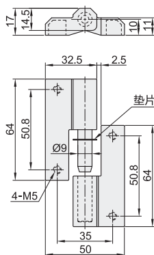
● 安装尺寸图
