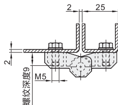
● 安装尺寸图
