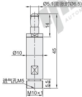
常规型 BWA01
