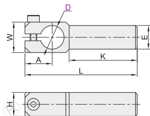
直杆型 BWA05
