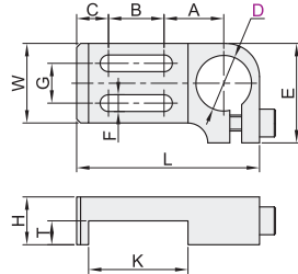
凹槽型 BWA04
