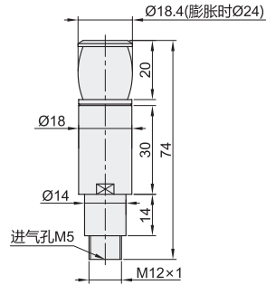
密闭型 BWA02
