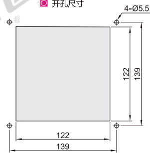
开孔尺寸
