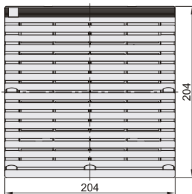
外形尺寸：9804
