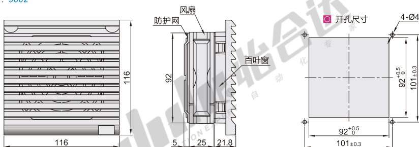
外形尺寸：9802
