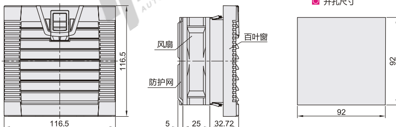
外形尺寸：9802H
