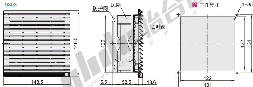
外形尺寸：9803
