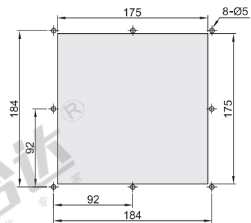
开孔尺寸
