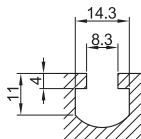
● 4080/8080槽口详图
